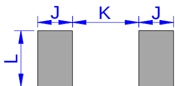
DO-214AB (SMC)
