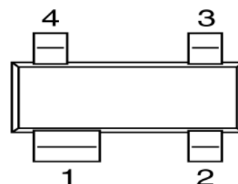
SOT143
