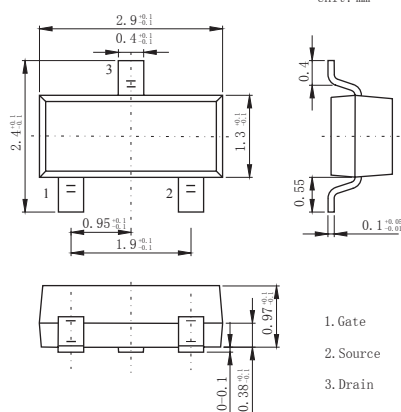
SOT-23
