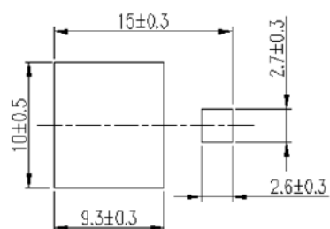
贴装端布局及尺寸
