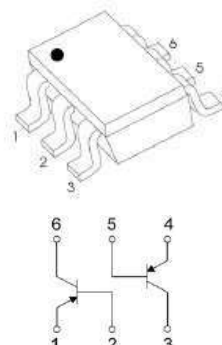
SOT-363
