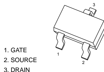
SOT-323
